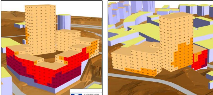
Maximal ljudnivå vid fasad, frifältsvärde. Vy från nordväst och från sydost. Bilder: ÅF
