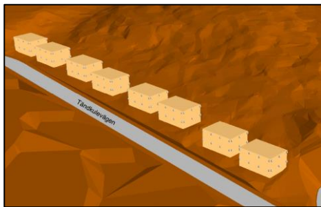
Maximal ljudnivå vid fasad, frifältsvärde. Vy från sydost och från nordväst. Bilder: ÅF
