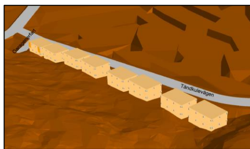
Maximal ljudnivå vid fasad, frifältsvärde. Vy från sydost och från nordväst. Bilder: ÅF
