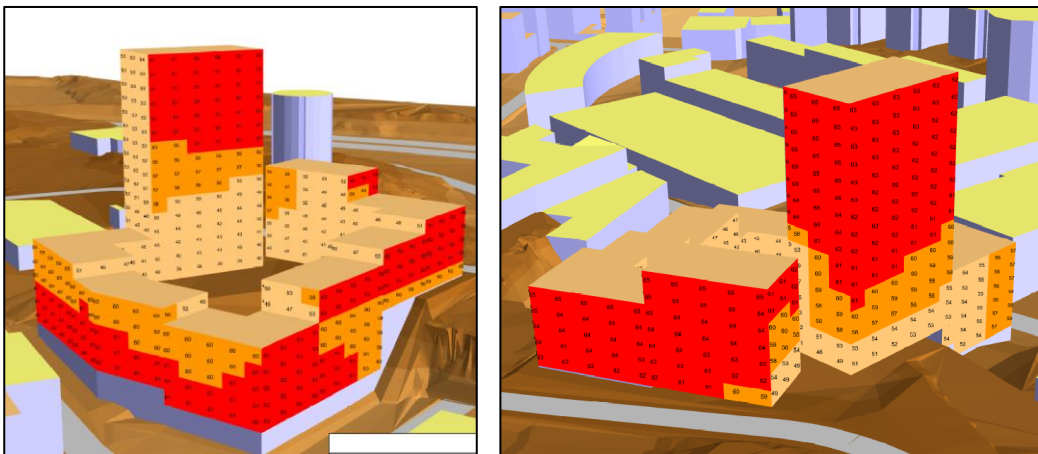
Ekvivalent ljudnivå vid fasad, frifältsvärde. Vy från nordväst och från sydost. Bilder: ÅF
