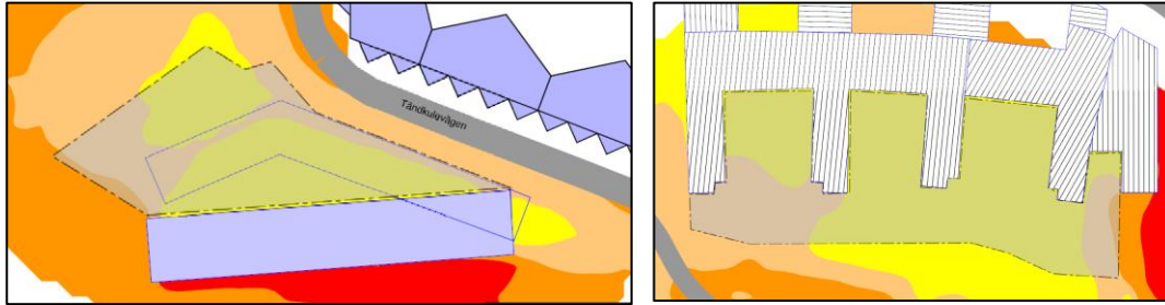
Dygnsequivärent ljudnivå vid förskola/förskolegård samt skolgård söder om hus 9. Bilder: ÅF
